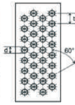
Trous ronds en lignes alternantes
