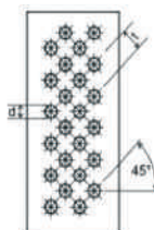
Trous ronds en lignes diagonalement alternantes
