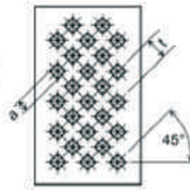
Quadratlochung in diagonal versetzten Reihen
