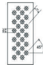
Rundlochung in diagonal versetzten Reihen
