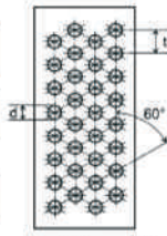
Rundlochung mit versetzten Reihen
